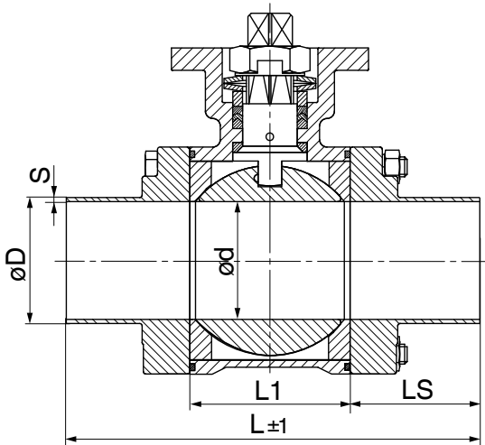
Spigots ASME code 59
